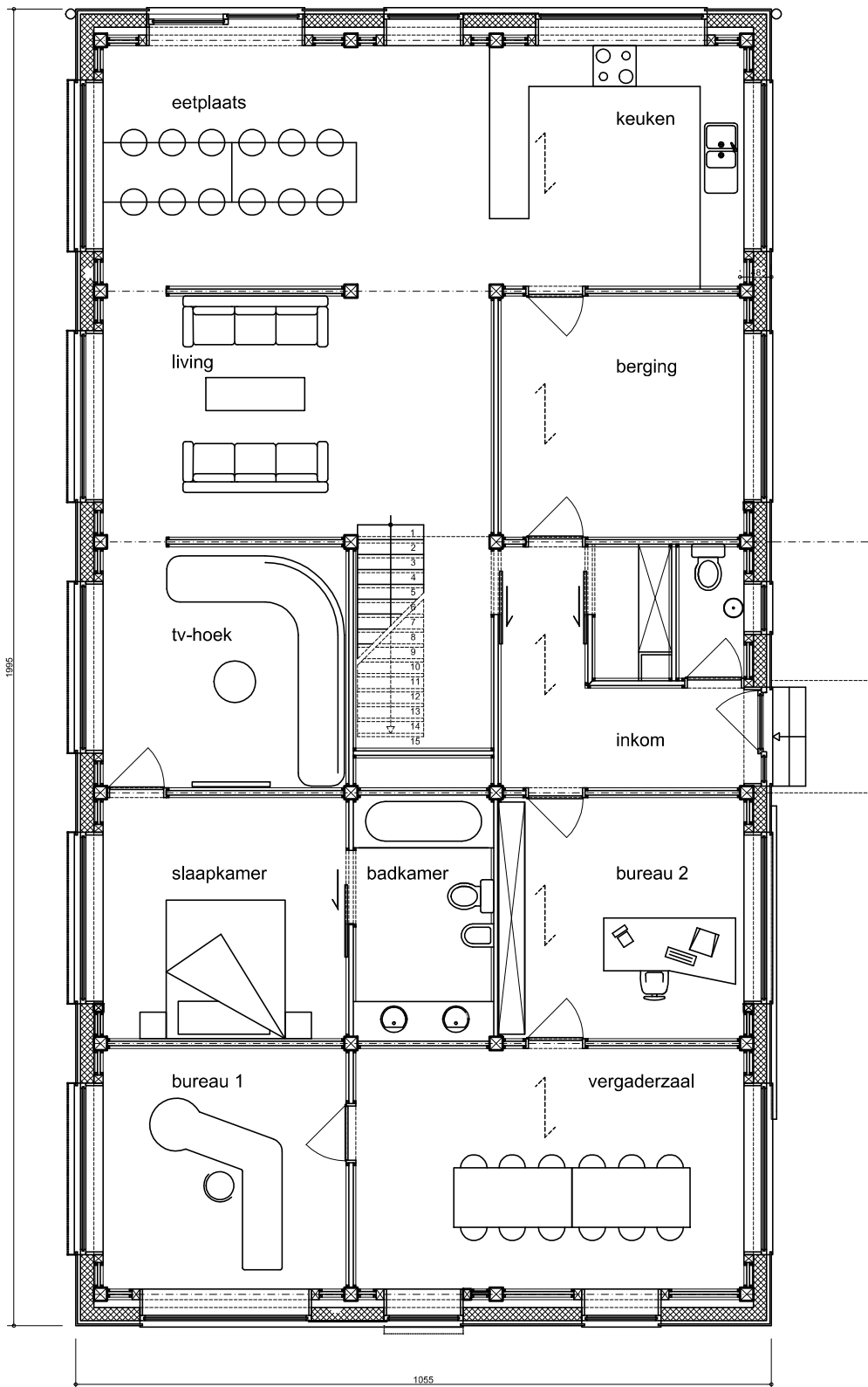
NIVEAU 0
